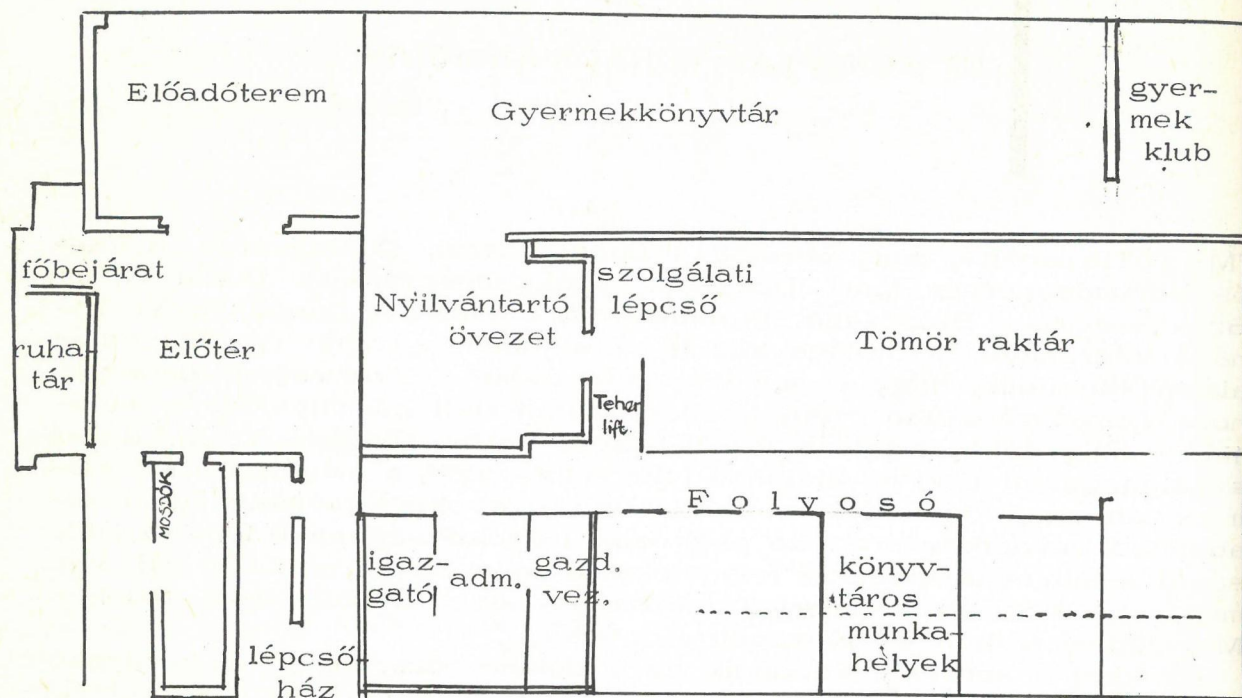
A könyvtár földszinti alaprajza
